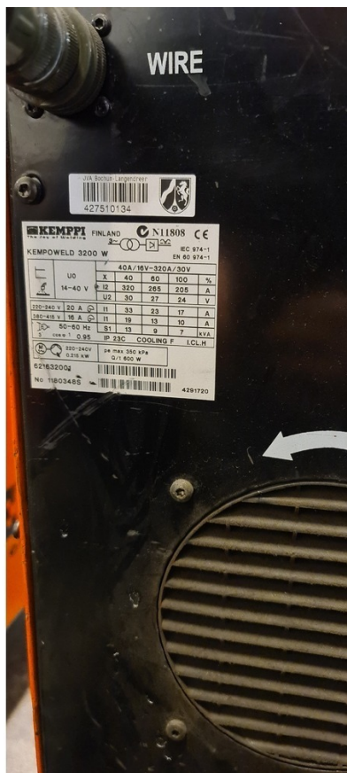
Bildbeschreibung: MIG / MAG Typenschild 2
