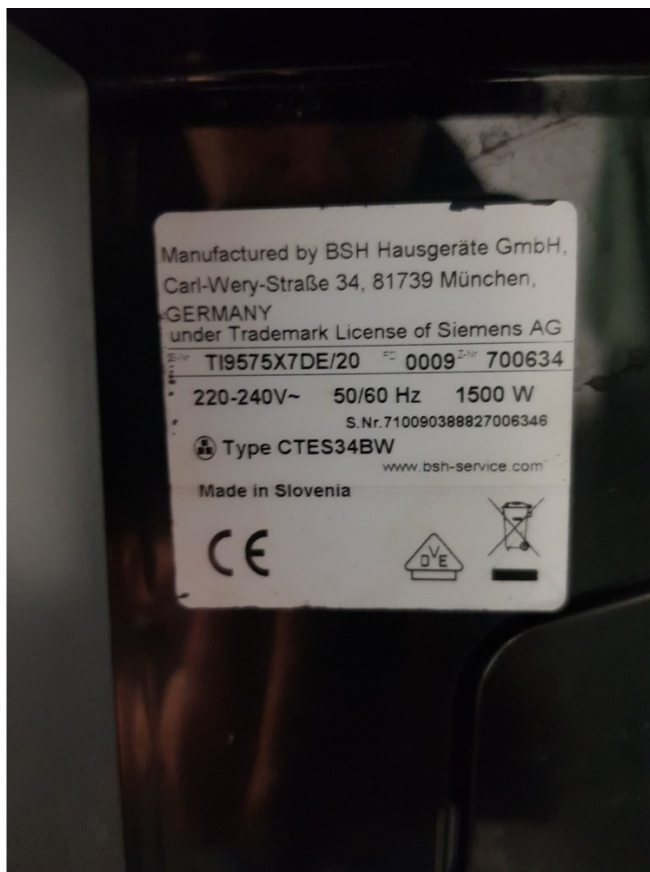
Bildbeschreibung: Typenschild
