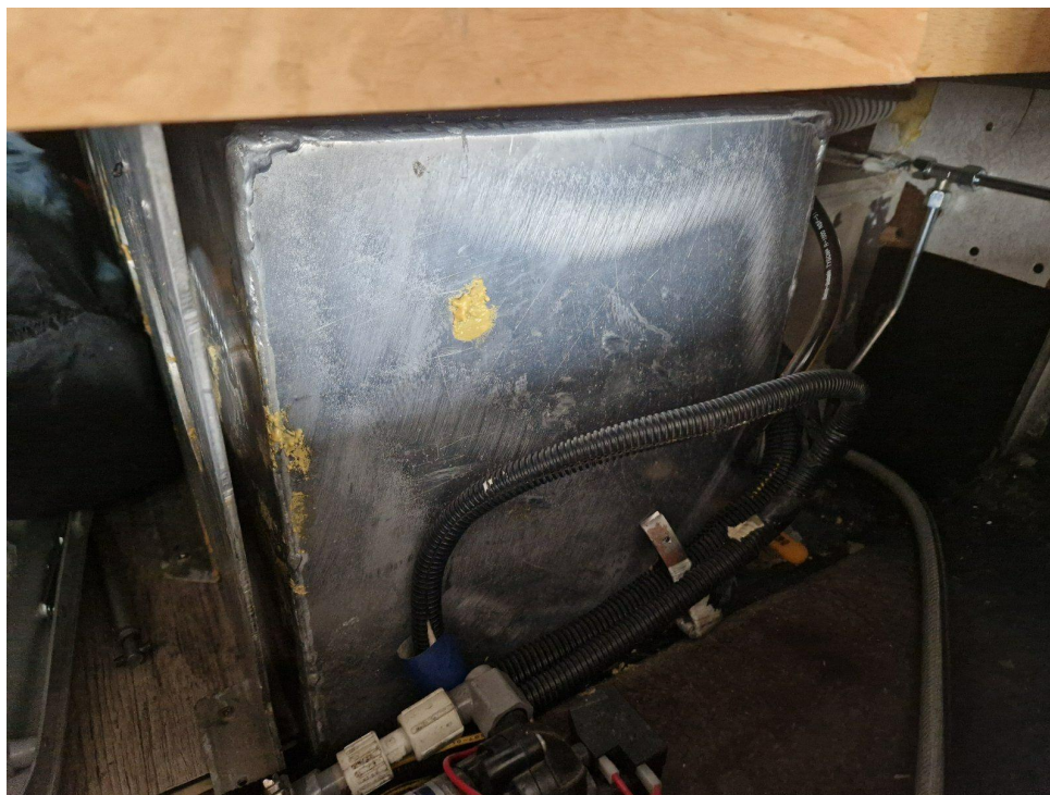
Bild 12 : Warmwasserspeicher
