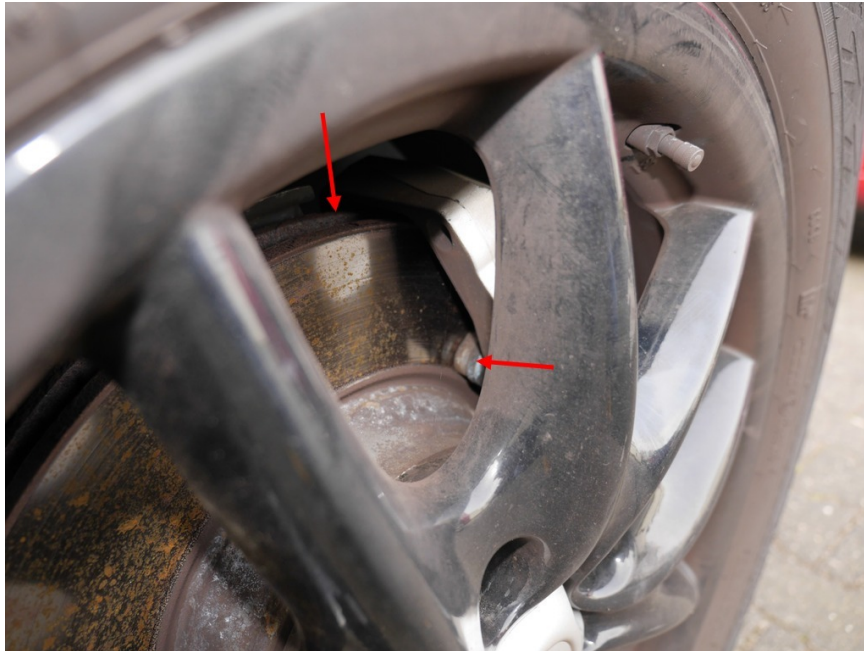
Bild 33 - Ausreichender Zustand der Bremsanlage
