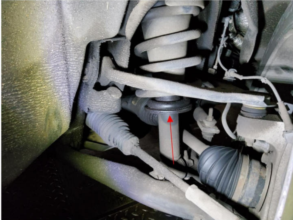
Bild 9 : Fahrwerk, Olverlust an vorderen Stoßdämpfern
