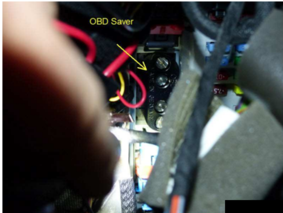
Bild 3 OBD Saver 2 eingebaut
