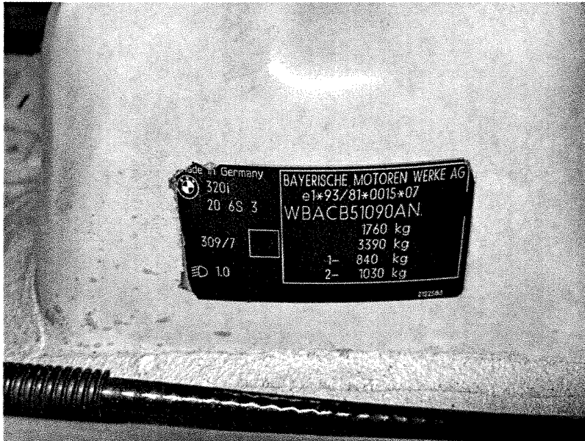
Fahrzeug-Identifizierungsnummer
