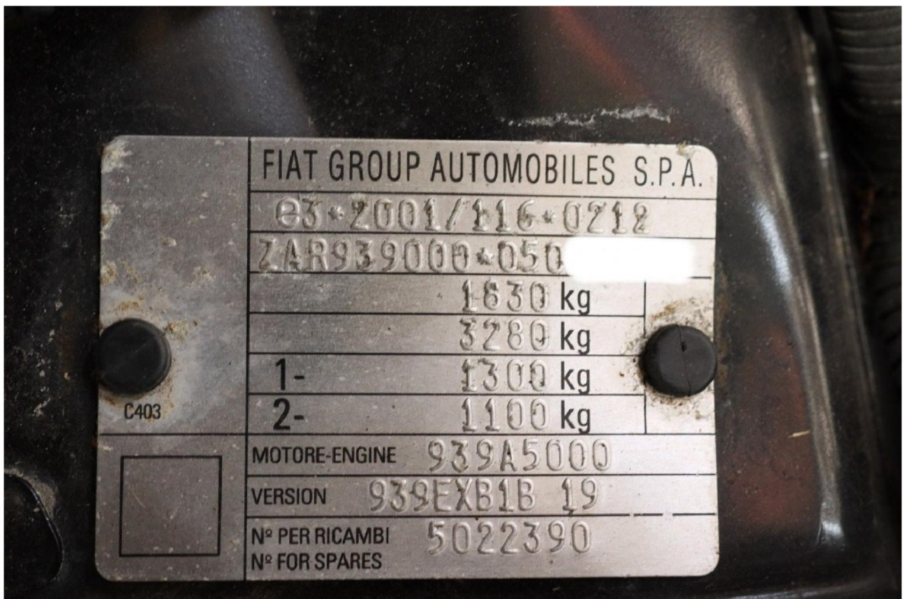
Bild 30: Fahrzeugidentifikationsnummer
