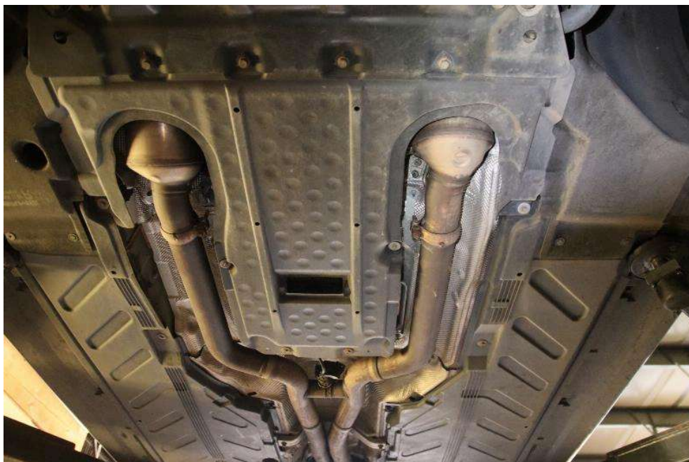
Bild: 40 Ansicht Unterboden mitte
