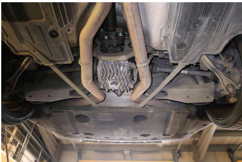
Bild: 42 Ansicht Unterboden hinten
