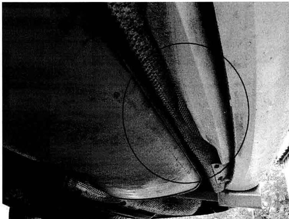
Bild 12 : Hitzeschutzblech hinten verformt
