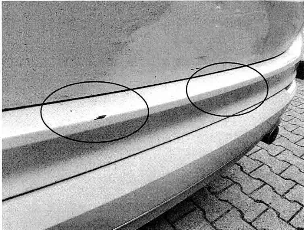
Bild 11 : Stoßfänger hinten Ladekante verschrammt
