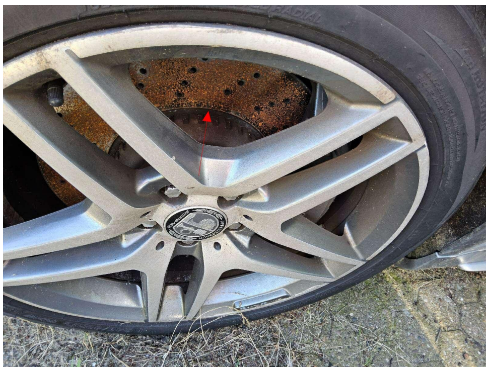
Bild 16 : Bremsanlage korrosionsgeschädigt
