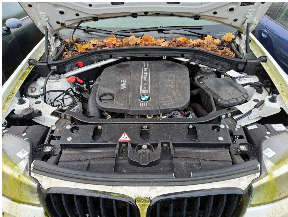
Bild 6 : Motorraum
