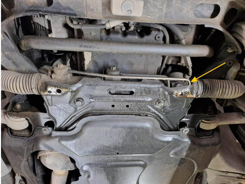
Bild 13 : Lenkgetriebe, Ölverlust am hydraulischen Anschluss
