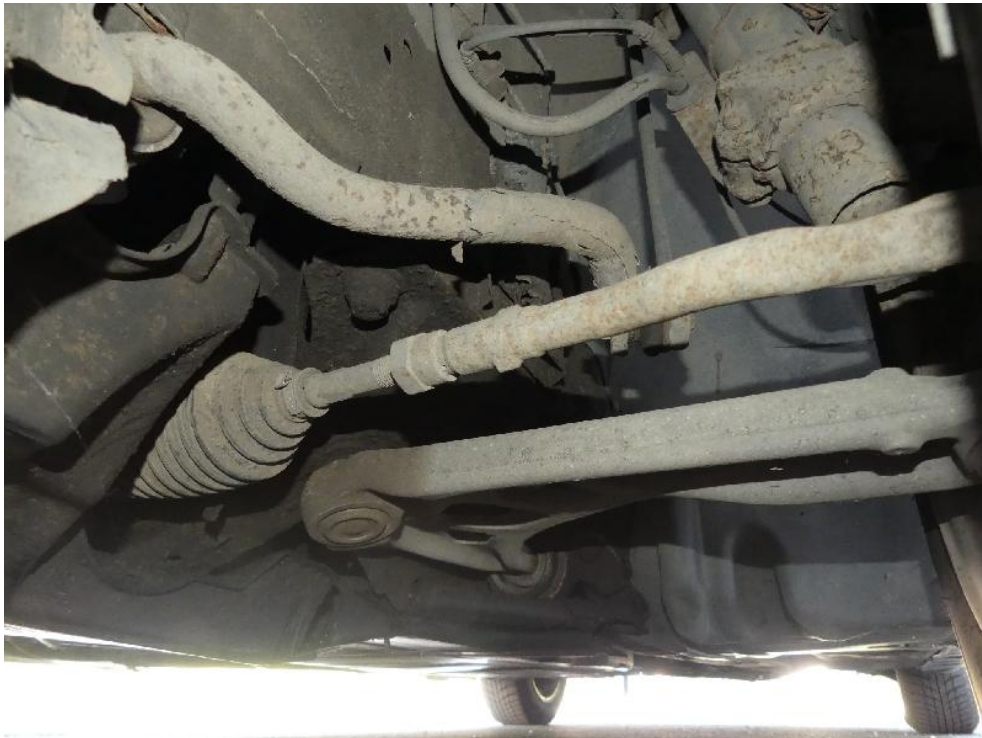
Bild: 87 Ansicht wie vor in geänderter Perspektive
