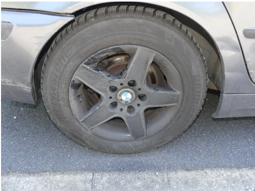
Bild: 58 Ausweisung der am Fahrzeug verbauten Rad/Reifenkombination hinten rechts.
