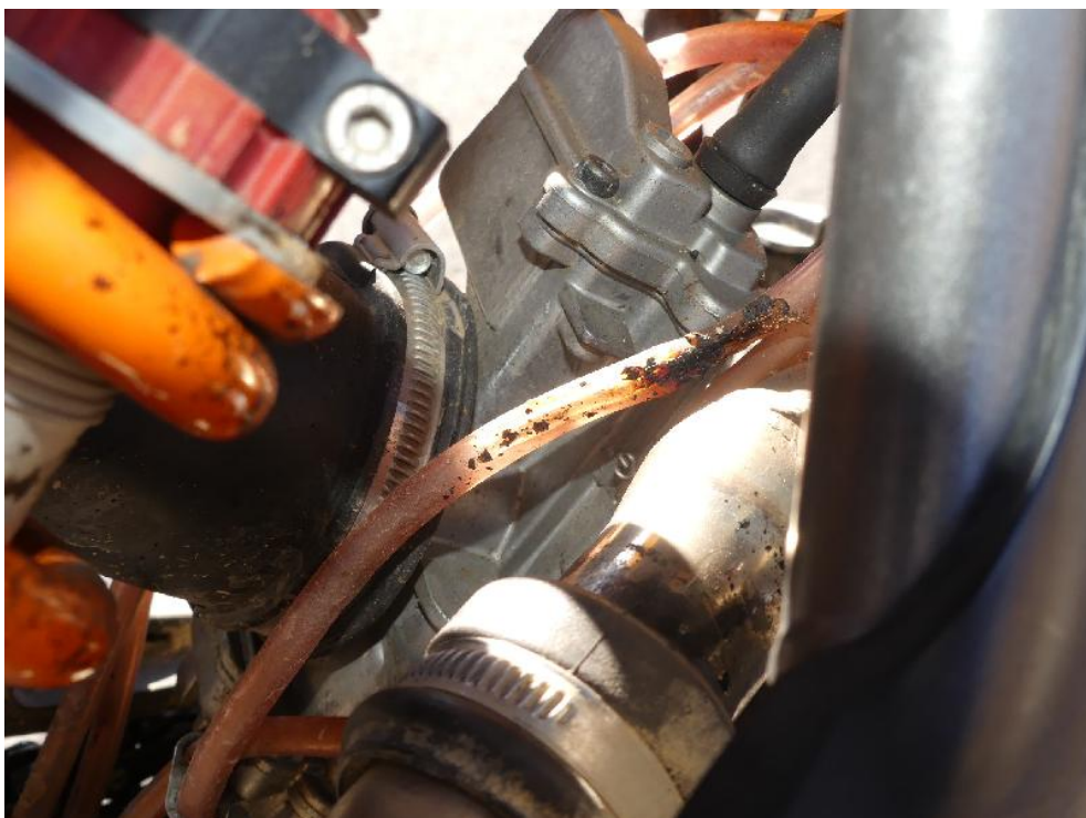
Bild: 38 Kraftstoffleitung liegt an der Abgasanlage an, diese ist partiell verschmolzen
