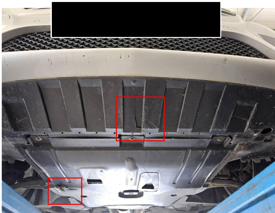
Bild 25 : Unterbodenverkleidung gebrochen
