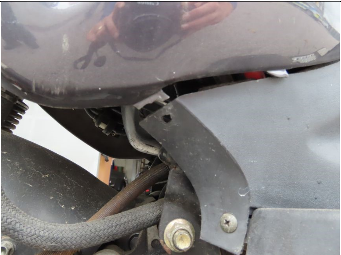
Bild 8 Verkleidung gebrochen
