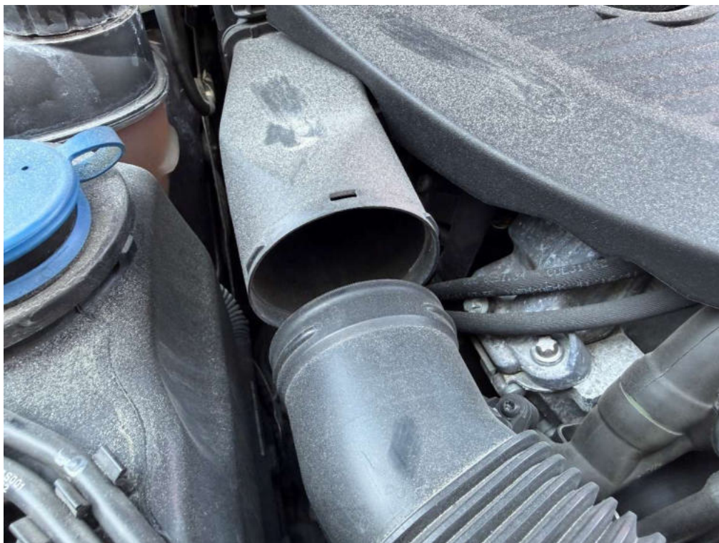
Bild 122 Detailaufnahme Lufteinlassschlauch beschädigt und Motorraum Sand und Staubablagerungen
