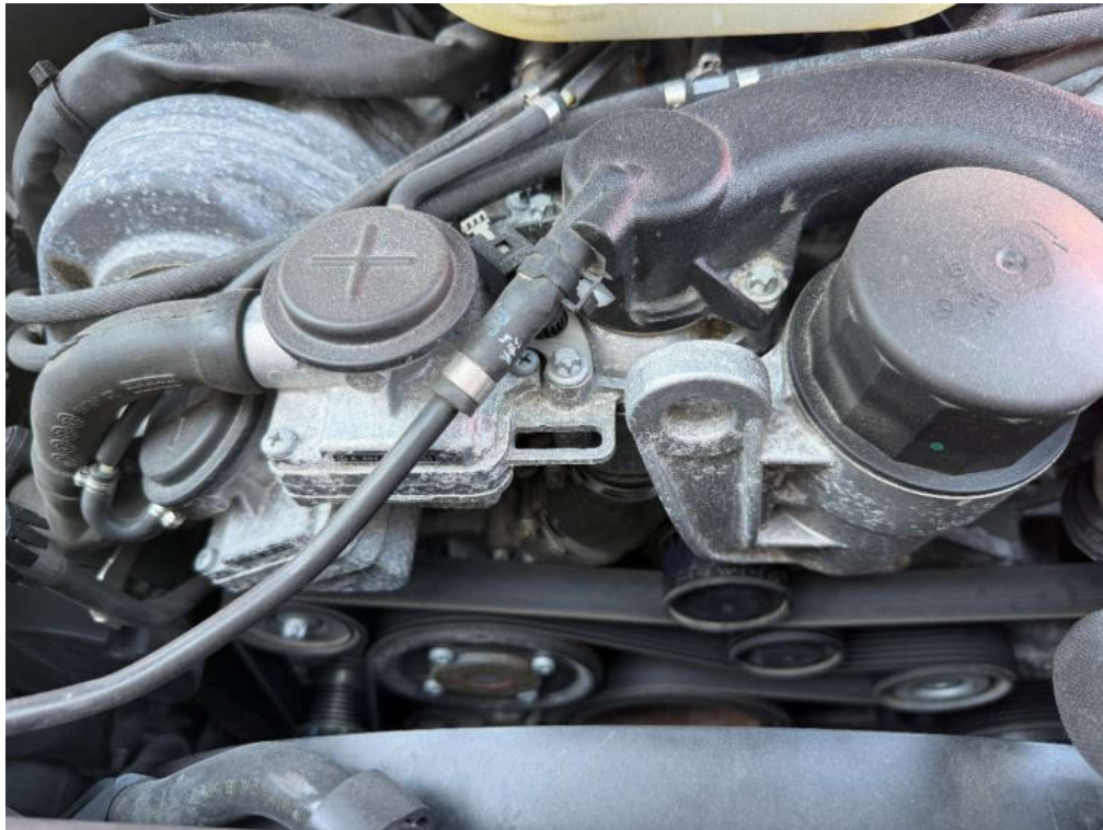
Bild 119 Detailaufnahme Ablagerungen an Nebenaggregaten
