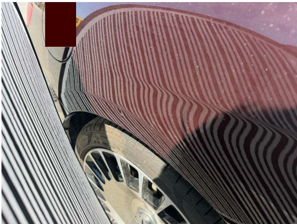
Bild 104 Detailaufnahme Seitenwand hinten rechts eingedellt
