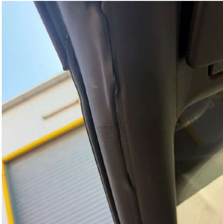
Bild 101 Detailaufnahme Verkleidung A-Säule und Dachhimmel beschädigt
