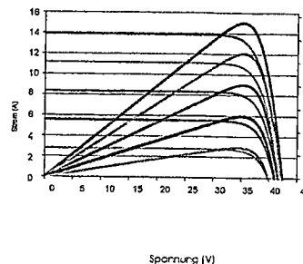
Strom-Spannungs- und Leistungs-Spannungs-Kennlinien (430 W)
