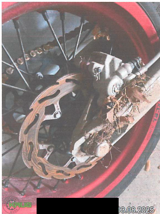
Foto 12: Bremsanlage hinten
