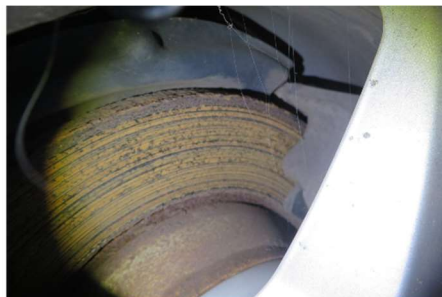
Bremsscheibe 2. Achse rechts
