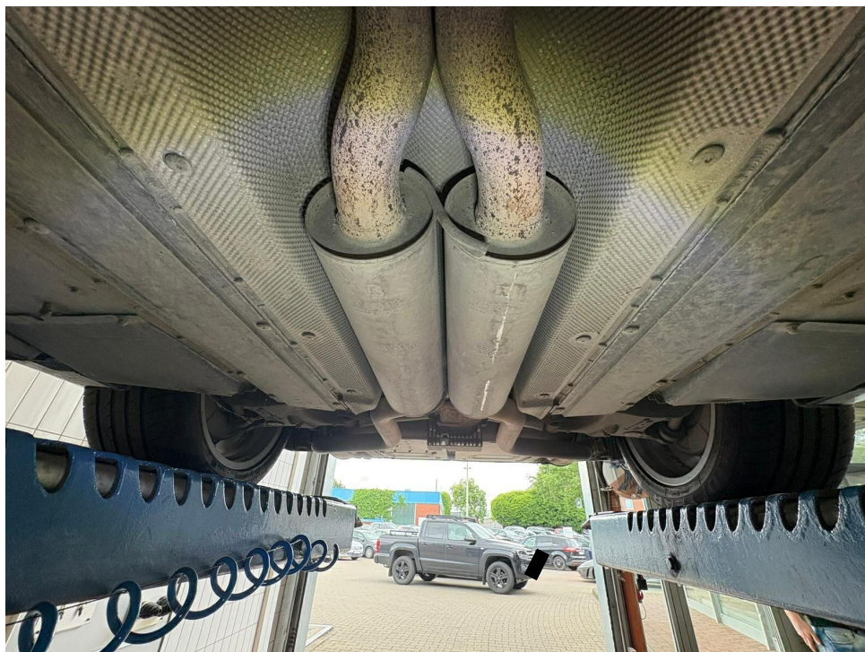
Bild 55 : Unterboden
