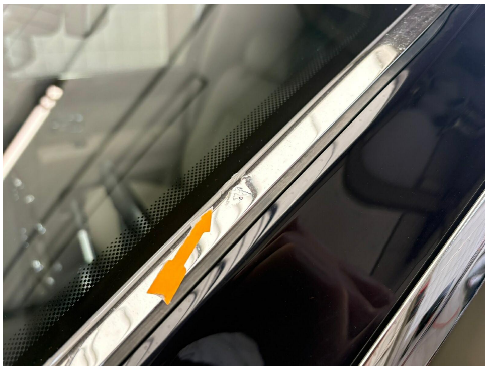
Bild 30 : Chromleiste Dachrahmen korrodiert
