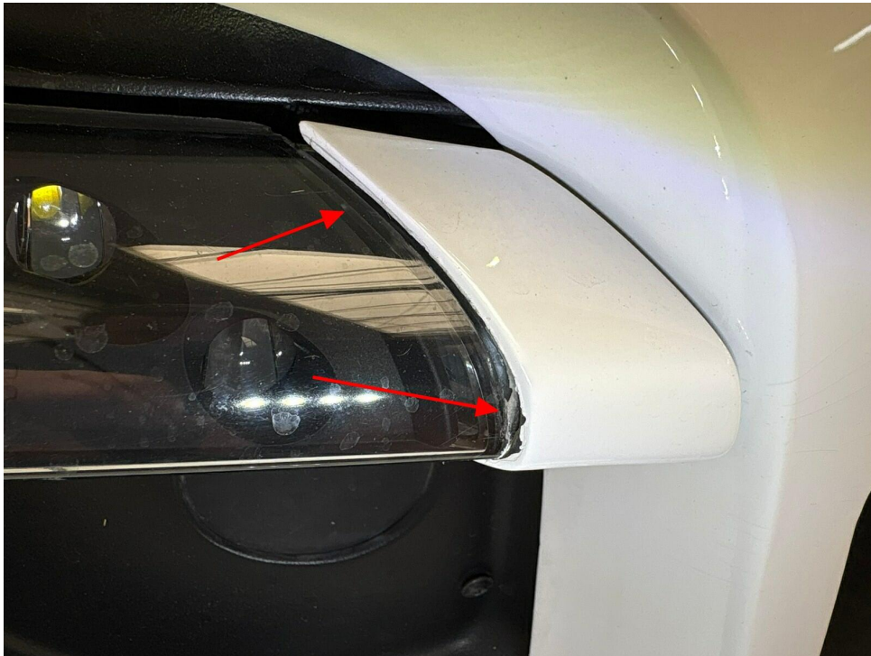
Bild 26 : Stossfänger vorne/Frontschürze Lackierung mehrfach gebrochen und unsachgemäß lackiert
