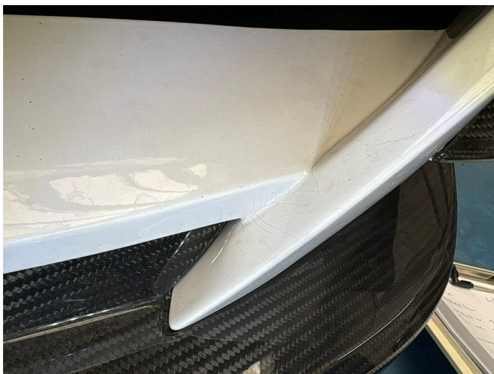
Bild 23 : Stossfänger vorne/Frontschürze Lackierung mehrfach gebrochen und unsachgemäß lackiert
