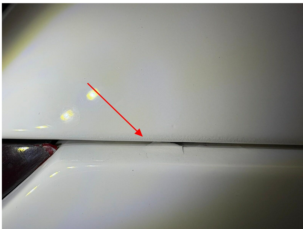
Bild 33 : Stossfänger hinten/Heckschürze Lackierung mehrfach gebrochen und unsachgemäß lackiert
