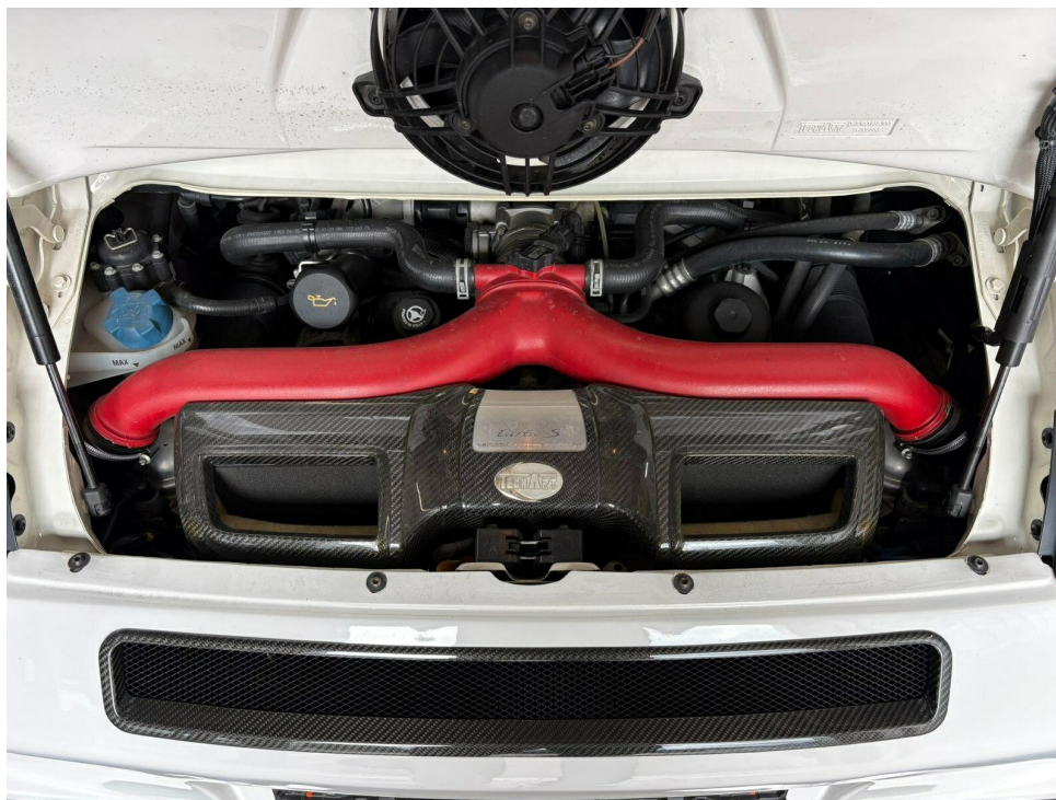
Bild 11 : Motorraum
