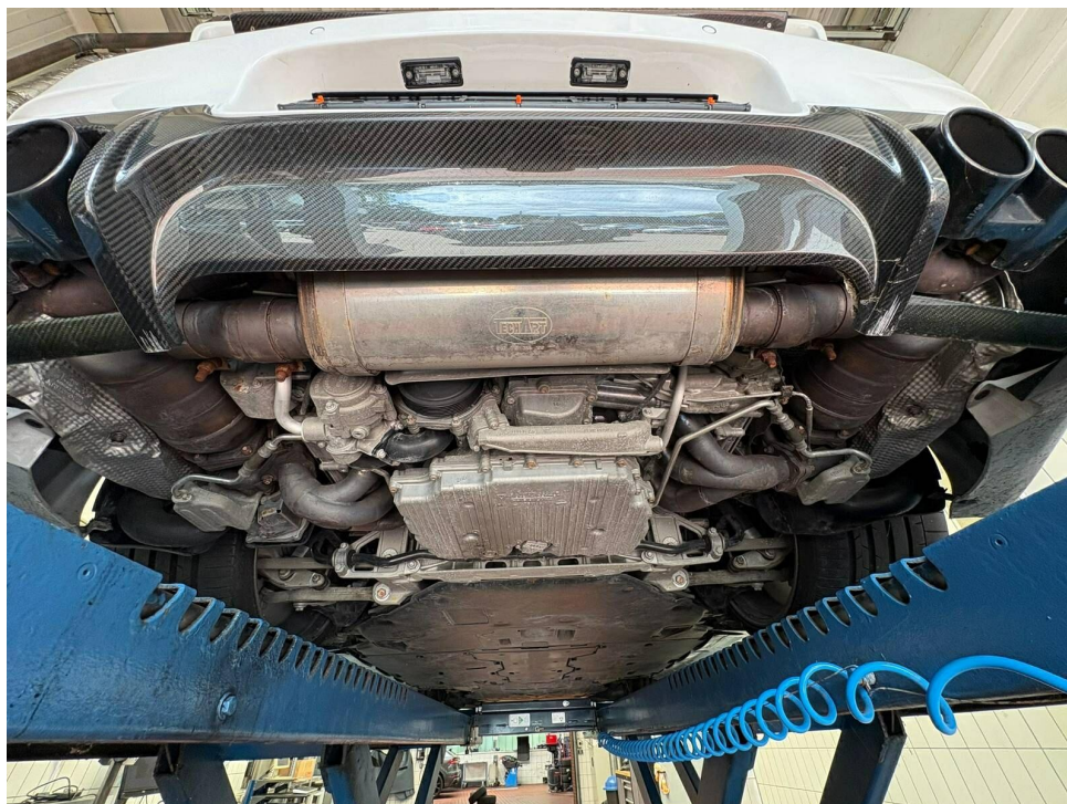
Bild 17 : Übersicht Motorraum unten
