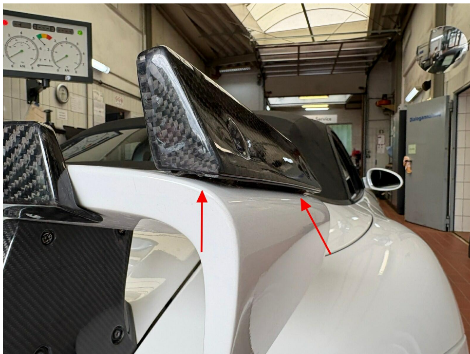
Bild 39 : Heckspoiler Carbon-Winglet rechts Befestigung lose
