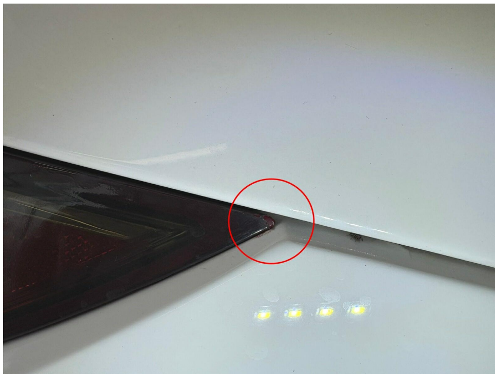
Bild 34 : Schlussleuchten rechts und links unsachgemäß foliert
