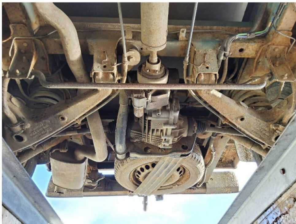
Bild 11 : Ansicht Unterboden, Berreich Hinterachse
