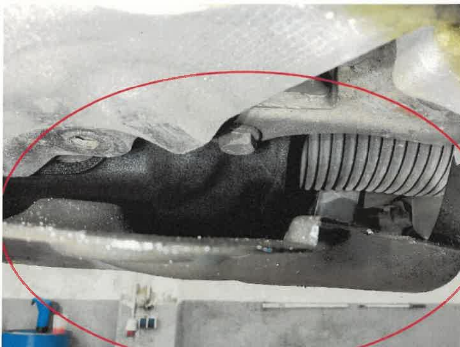
Bild 24 : Motorölverlust
