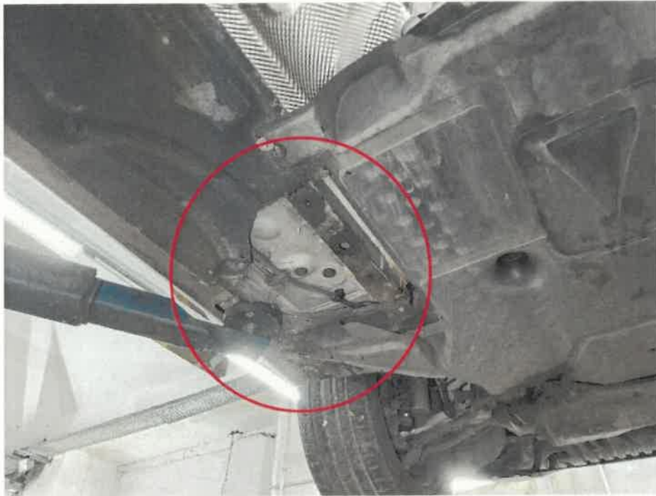
Bild 25 : Unterbodenverkleidung links gebrochen.
