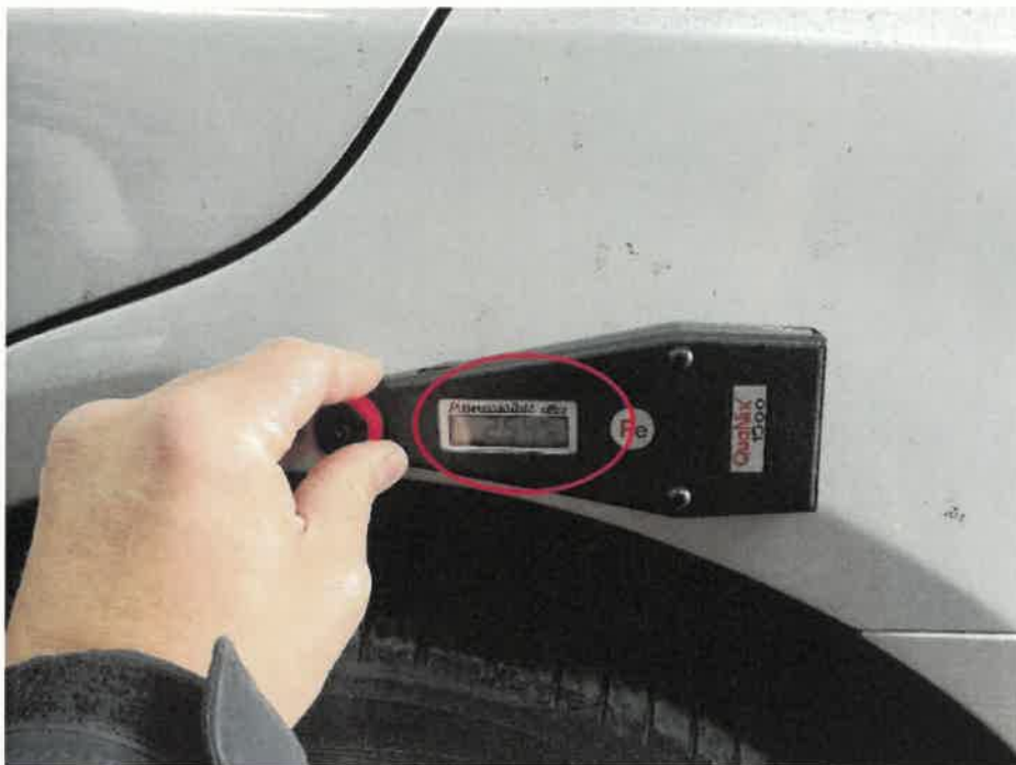
Bild 14 : gemessene Lackschichtdicke an der Seitenwand hinten links (2.540 \mu )
