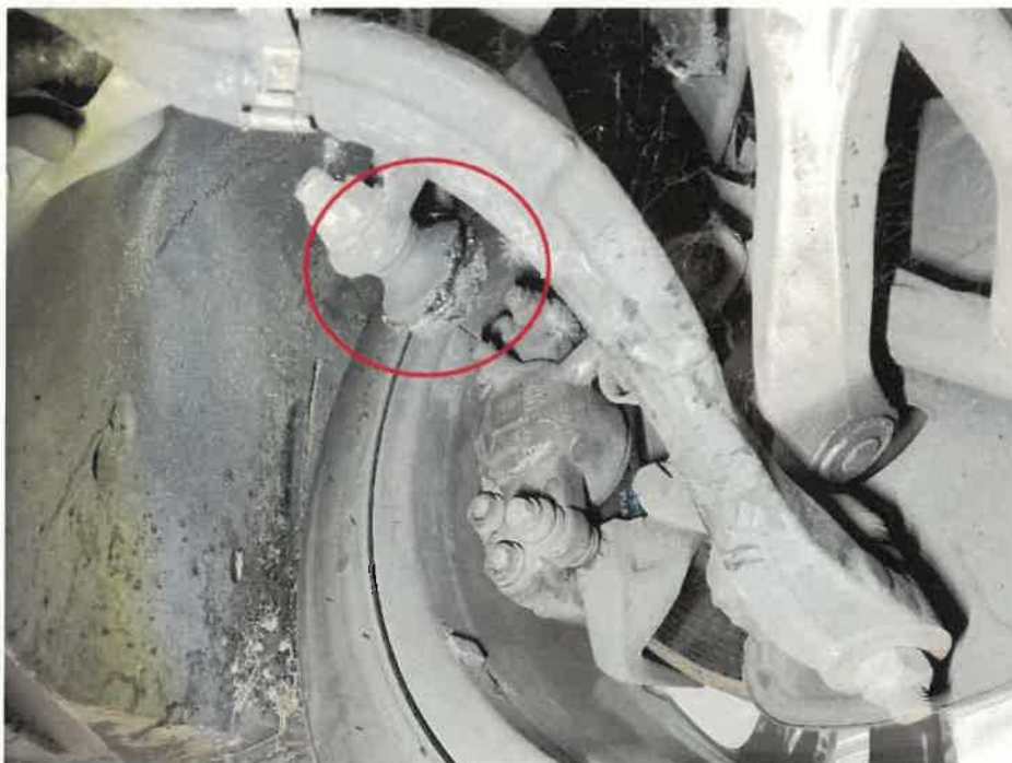
Bild 22 : Pendelstütze vorne links, Manschette eingerissen
