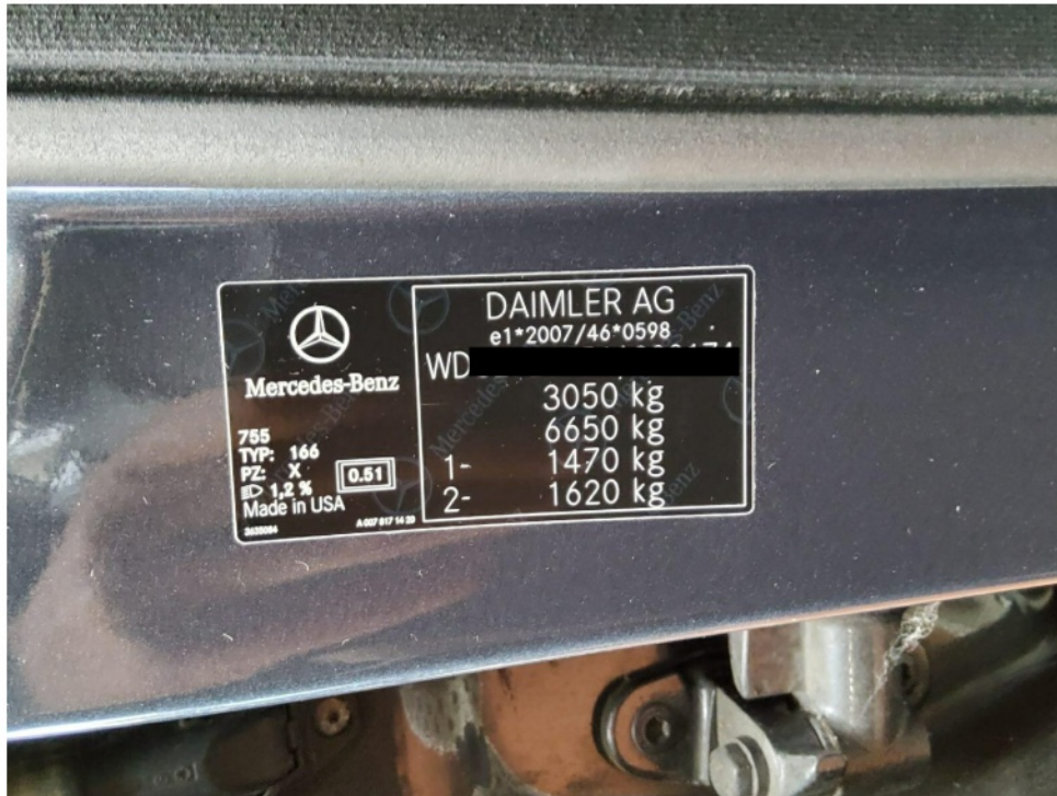
Bild 5 : Typschild
