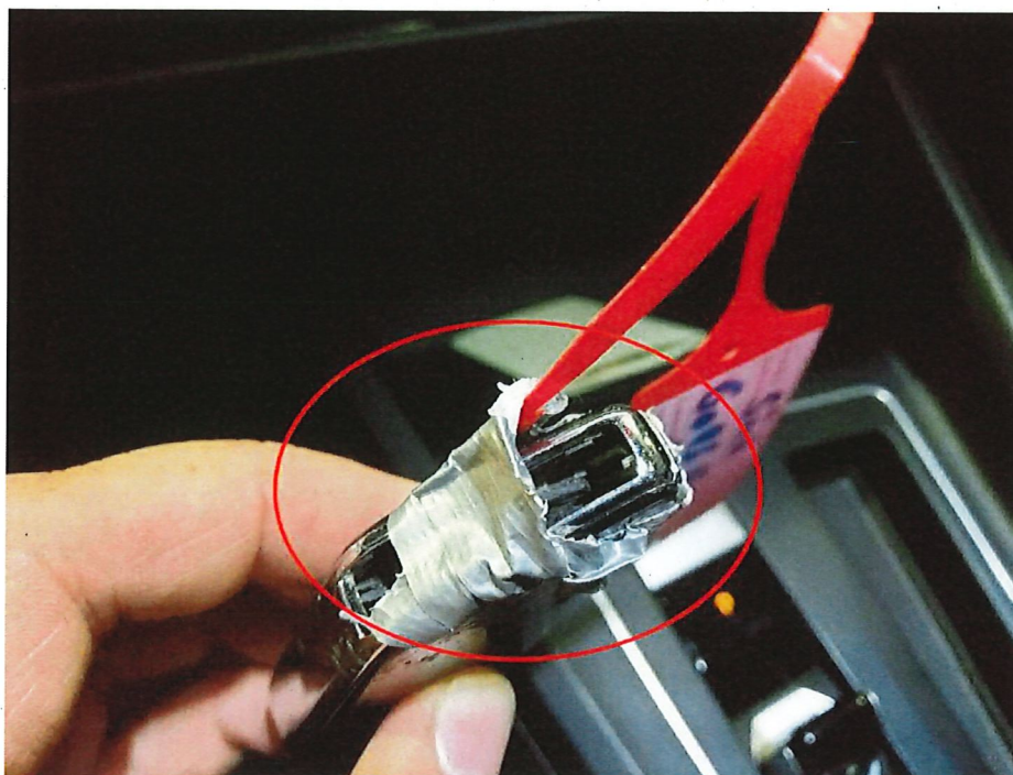
Bild 7 : Fahrzeugschlüssel gebrochen
