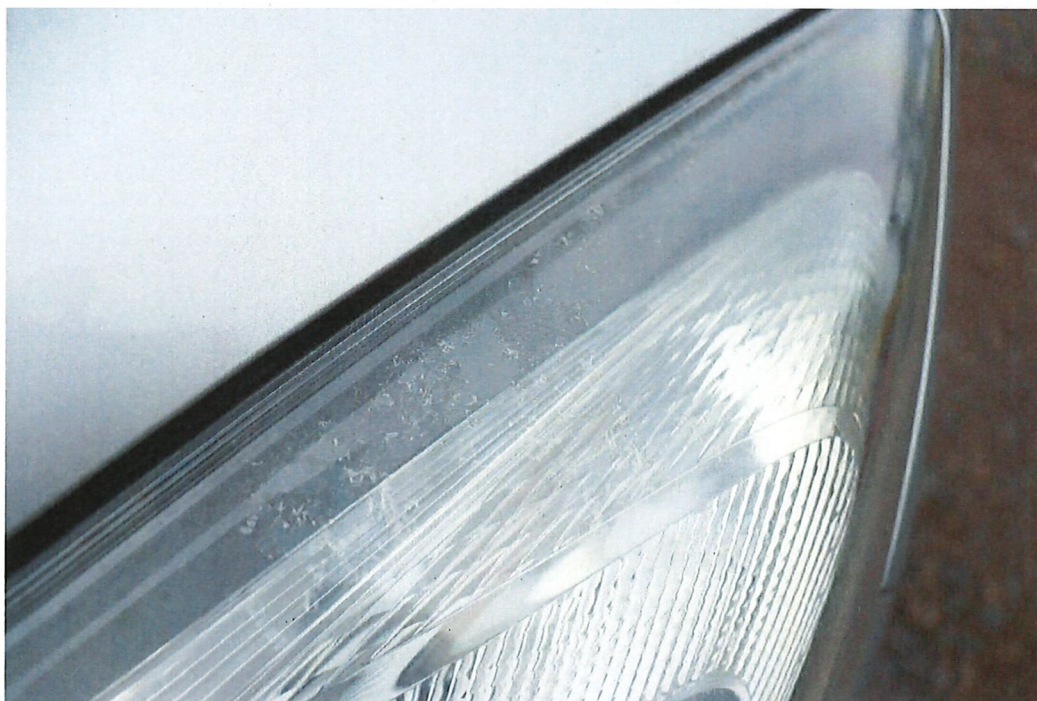
Bild 32 : Abblendlichtscheinwerfer links Ablösung des Kunststoffes
