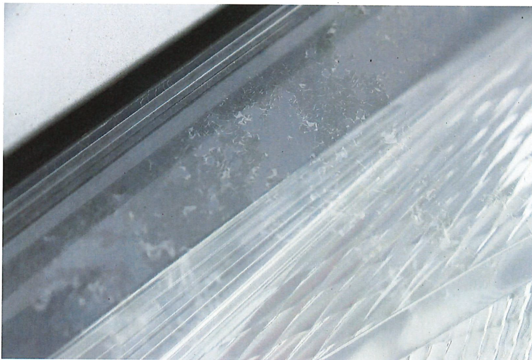
Bild 33 : Abblendlichtscheinwerfer links Ablösung des Kunststoffes
