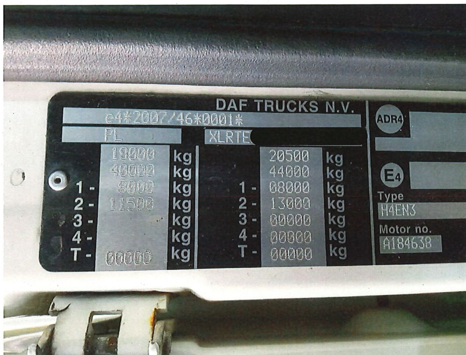
Bild 5 : Typenschild
