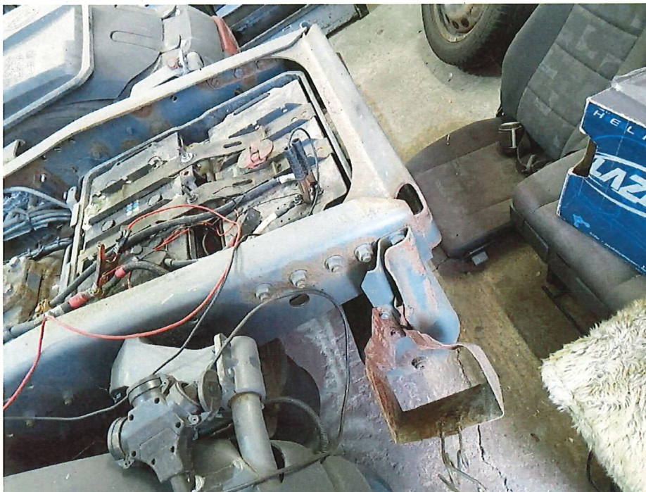
Bild 12 : Korrosion
