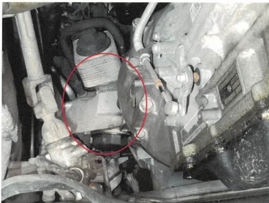
Bild 16 : Kühlwasserverlust
