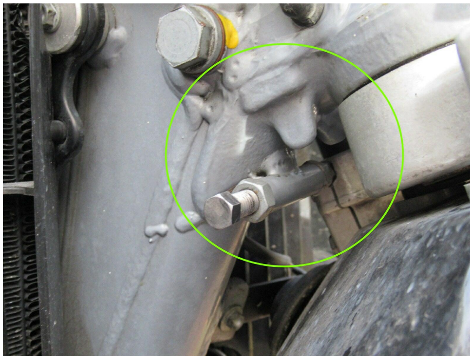
Bild 12 : Lenkanschlag intakt
