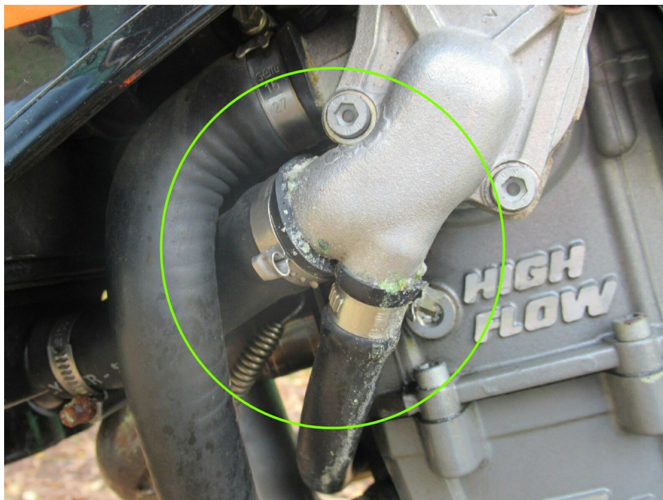
Bild 11 : Wasserverlust Thermostat
