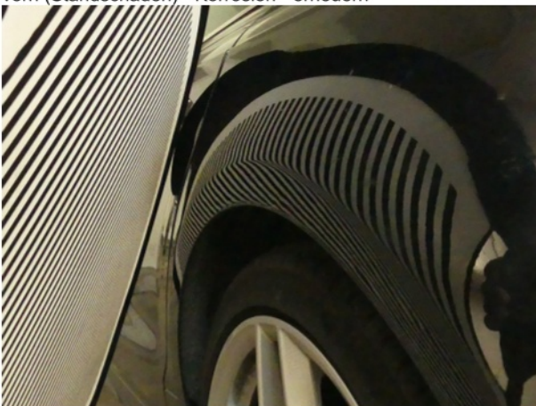
Beschädigung #17: Seitenwand links: Seitenwand (Wellig, Staubeinschlüsse) - nicht fachgerecht instandgesetzt -
