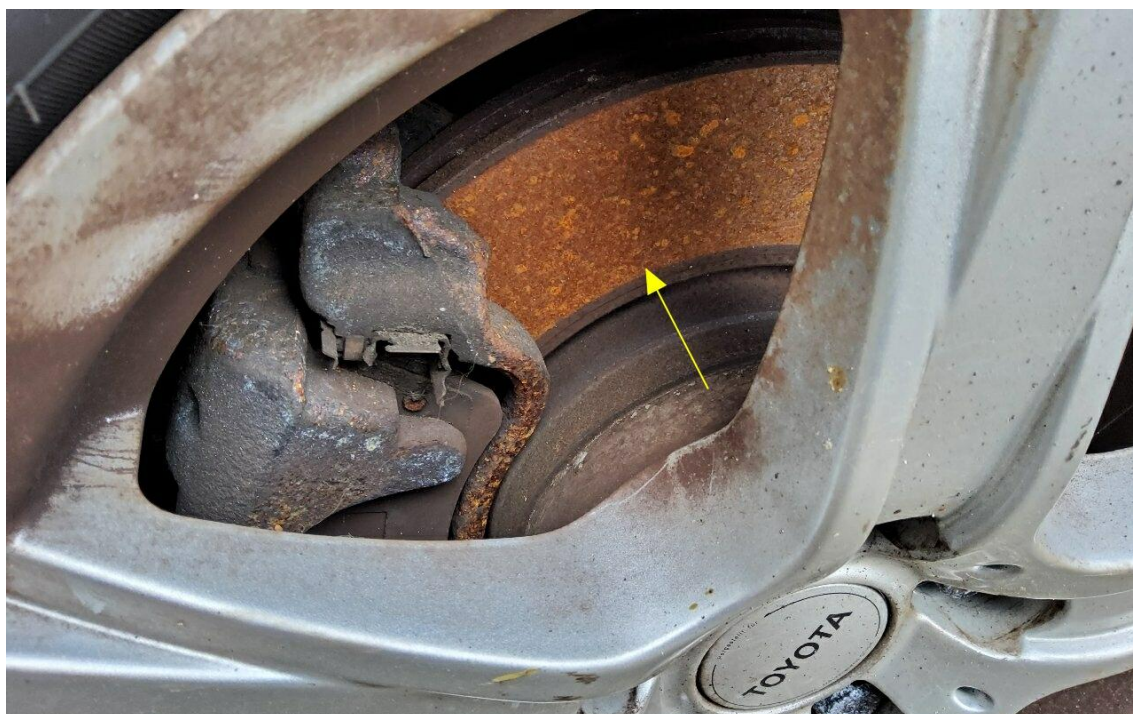
Bild 14 : Bremsscheiben vorne und hinten Tragbild mangelhaft
