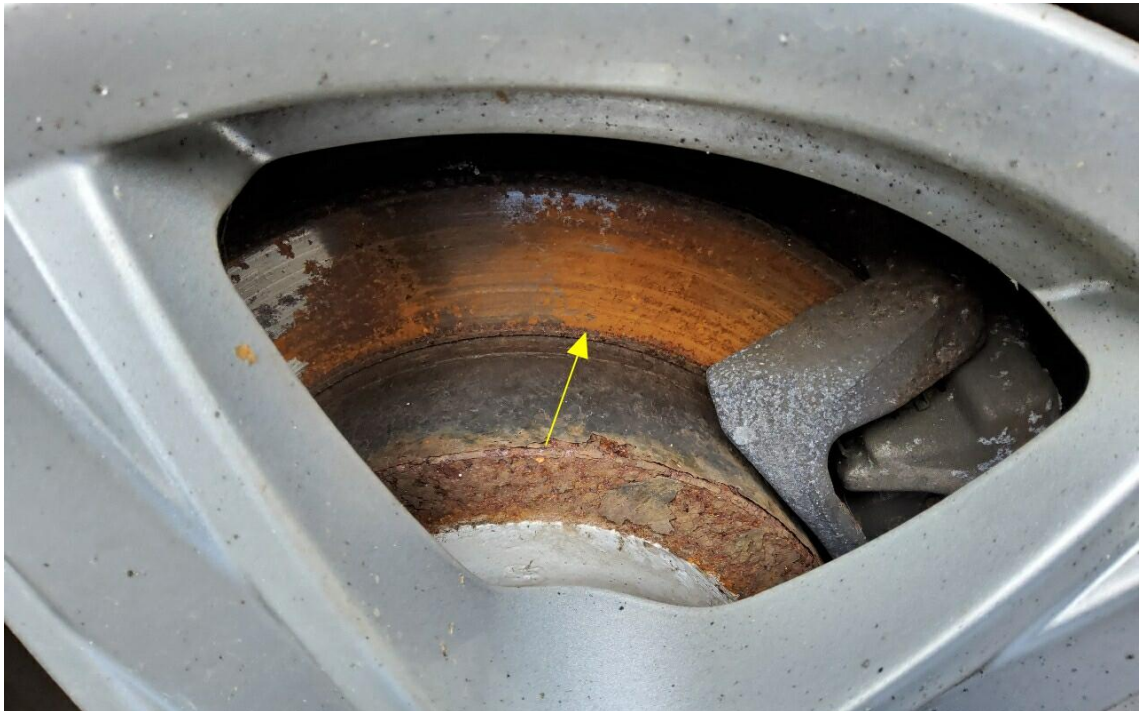
Bild 15 : Bremsscheiben vorne und hinten Tragbild mangelhaft
